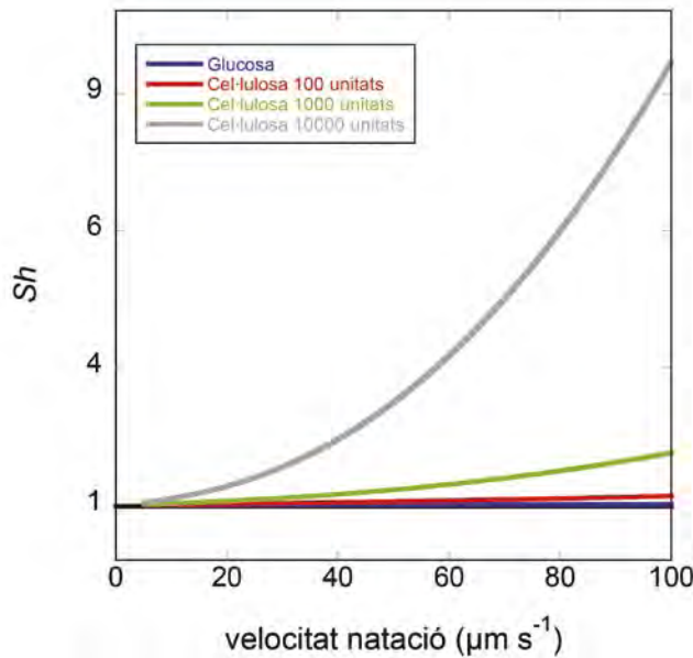
↑ Figura 2. Comportament del Sh amb la velocitat de natació d'un bacteri de 0,5 \mu\text{m} de diàmetre. Les línies corresponen a diferents compostos de creixent pes molecular i , per tant, de decreixent difusivitat. La línia horitzontal negra marca Sh = 1 (difusió molecular només).
