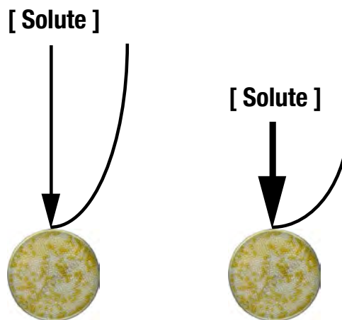
↑ Figura 1. Representació gràfica del gradient de la concentració d'un solut des del camp llunyà fins a la superfície d'un microorganisme. Si el camp llunyà és més a prop del microorganisme (dreta), el gradient del solut serà més gran i, per tant, també el flux cap a l'organisme.
