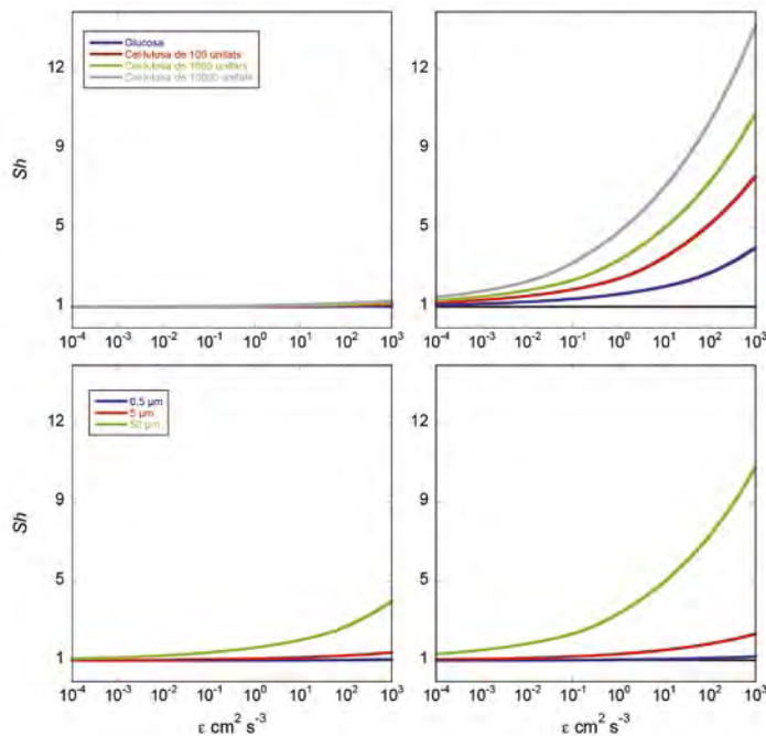
↑ Figura 3. Comportament del Sh amb la turbulència per a diferents compostos de creixent pes molecular i , per tant, de decreixent difusivitat (dalt) per a un microorganisme de 0,5 \mu\text{m} de diàmetre (dalt-esquerra) i 50 \mu\text{m} de diàmetre (dalt-dreta), i per a diferents mides de microorganismes (baix) per a glucosa (baix-esquerra) i per a cel·lulosa de 1.000 monòmers (baix-dreta). La línia horitzontal negra marca Sh = 1 (difusió molecular només).
